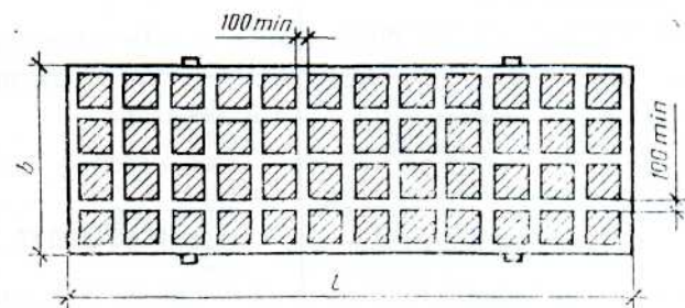
Расположение нагрузки на плите в плане
