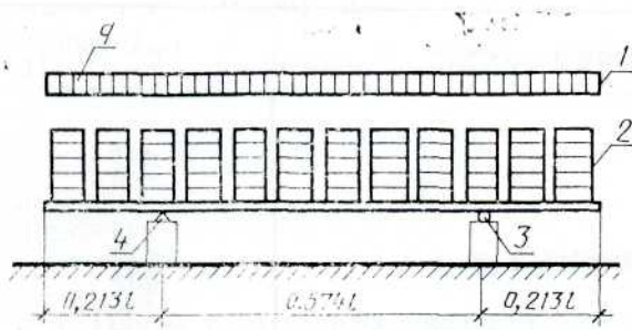
Схема опирания плиты
